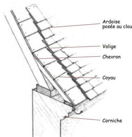
Clouage à 1 clou
